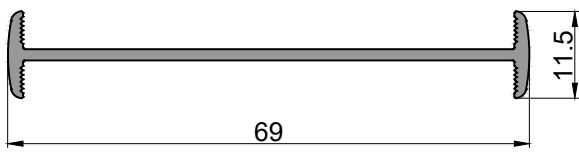
1165 Unionero 64mm 2.190 kg/tira Largo: 6020 mm
