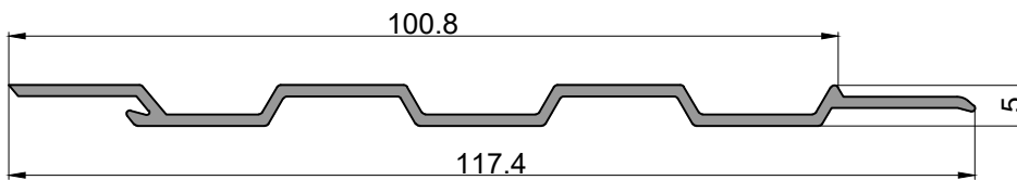
992 Revestimiento acanalado 3.990 kg/tira Largo: 6020 mm Bonificado
